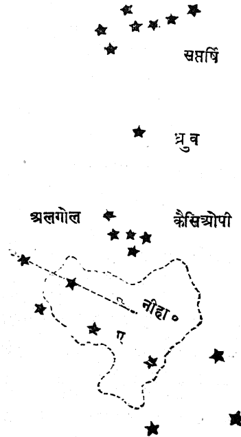
चित्र ५—एयड्रोमीडा नीहारिका
